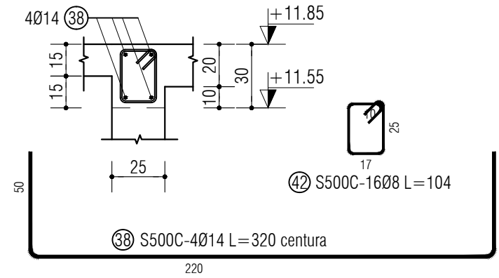
Sectiunea 6-6 perete P1 1 buc. - scara 1:25
