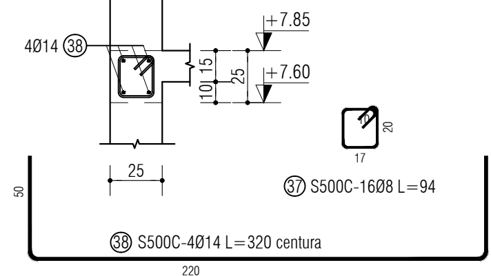
Sectiunea 4-4 perete P1 1 buc. - scara 1:25
