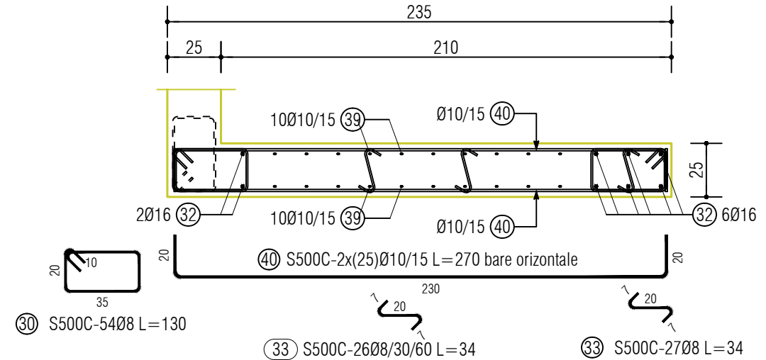
Sectiunea 1-1 perete P2 1 buc. - scara 1:25
