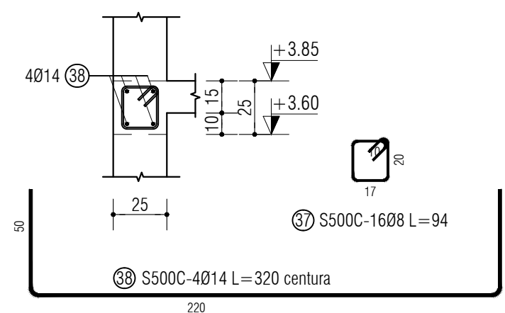
Sectiunea 1-1 perete P1 1 buc. - scara 1:25
