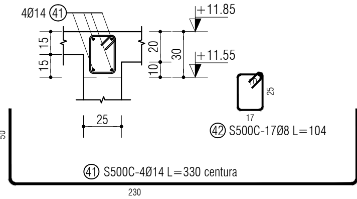
Sectiunea 6-6 perete P2 1 buc. - scara 1:25
