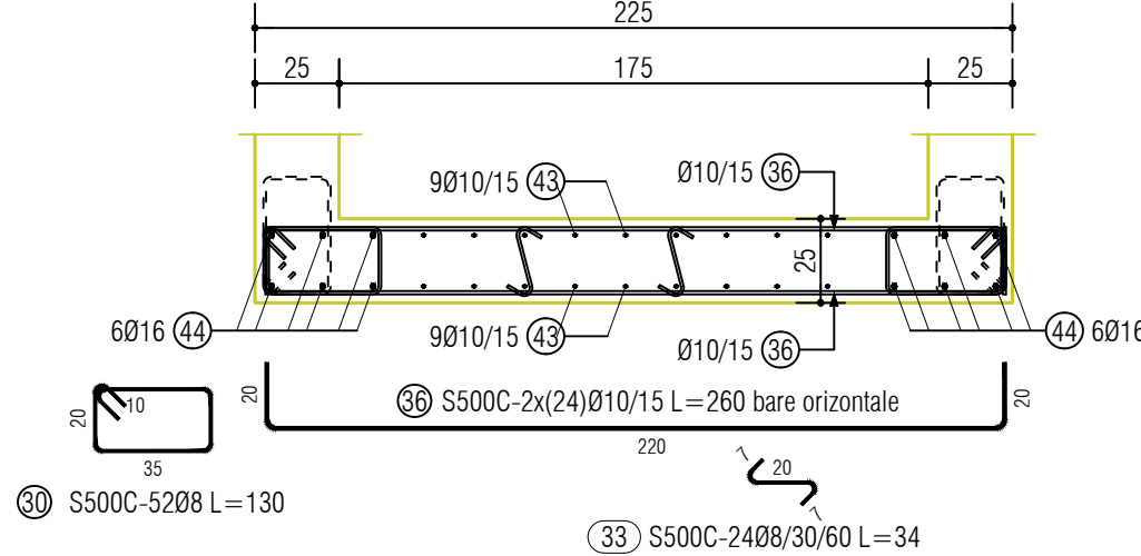
Sectiunea 3-3 perete P1 1 buc. - scara 1:25
