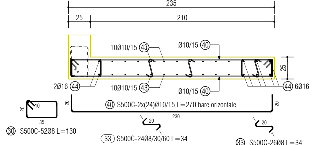
Sectiunea 3-3 perete P1 1 buc. - scara 1:25
