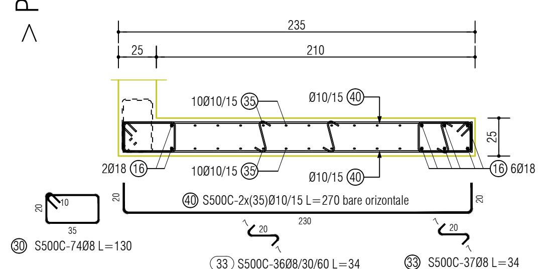
Sectiunea 2-2 perete P2 1 buc. - scara 1:25
