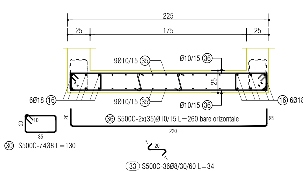
Sectiunea 2-2 perete P1 1 buc. - scara 1:25
