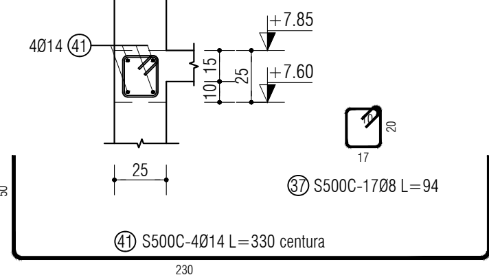
Sectiunea 4-4 perete P2 1 buc. - scara 1:25
