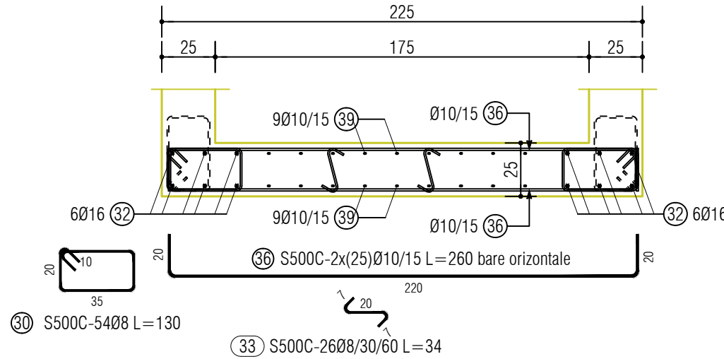
Sectiunea 4-4 perete P1 1 buc. - scara 1:25
