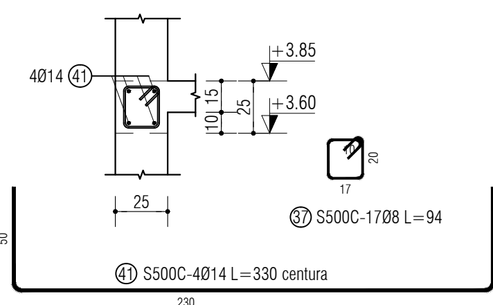
Sectiunea 2-2 perete P2 1 buc. - scara 1:25
