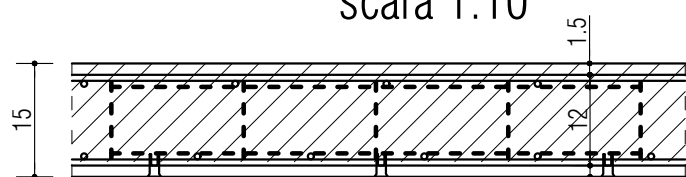
DETALIU DISTANTIER MONTARE ARMATURI scara 1:10
