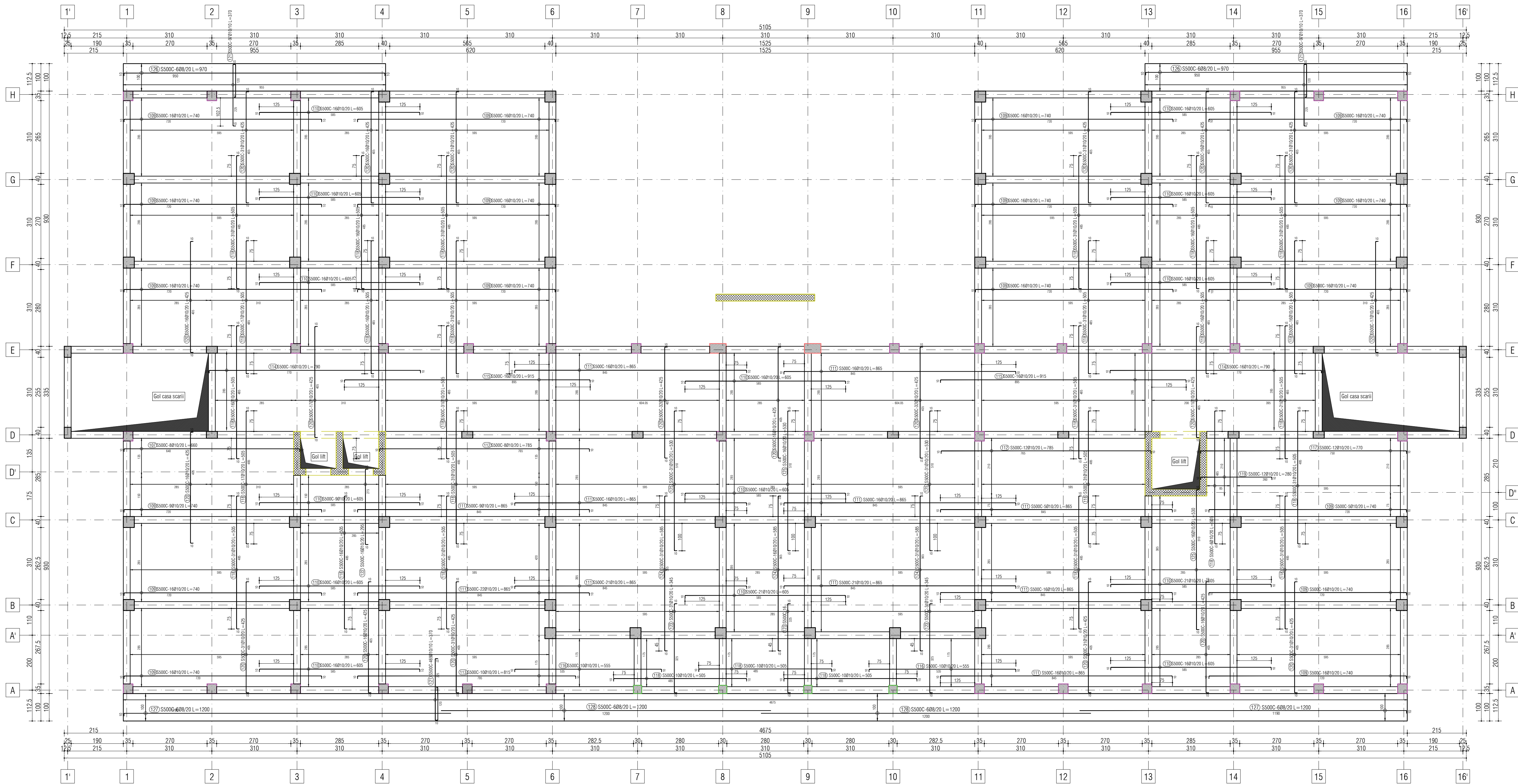
PLAN ARMARE SUPERIOARA PLANSEU PARTER scara 1:75
