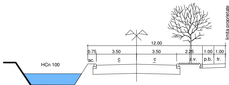
PROFIL TRANSVERSAL TIP - 12 M - PTT4
