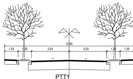
PROFIL TRANSVERSAL TIP - 12 M -
