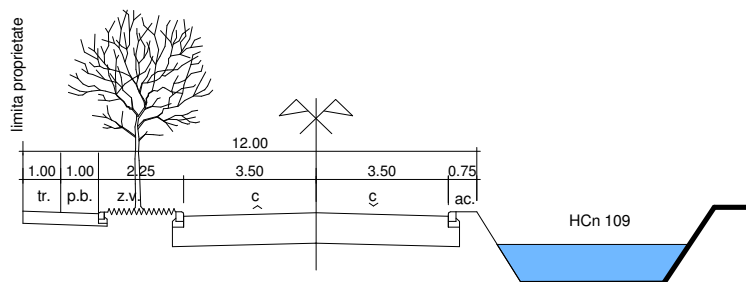
PROFIL TRANSVERSAL TIP - 12 M - PTT3
