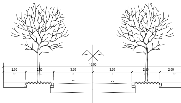
PROFIL TRANSVERSAL TIP - 16 M - PTT2
